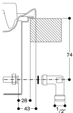
Газовое подключение
